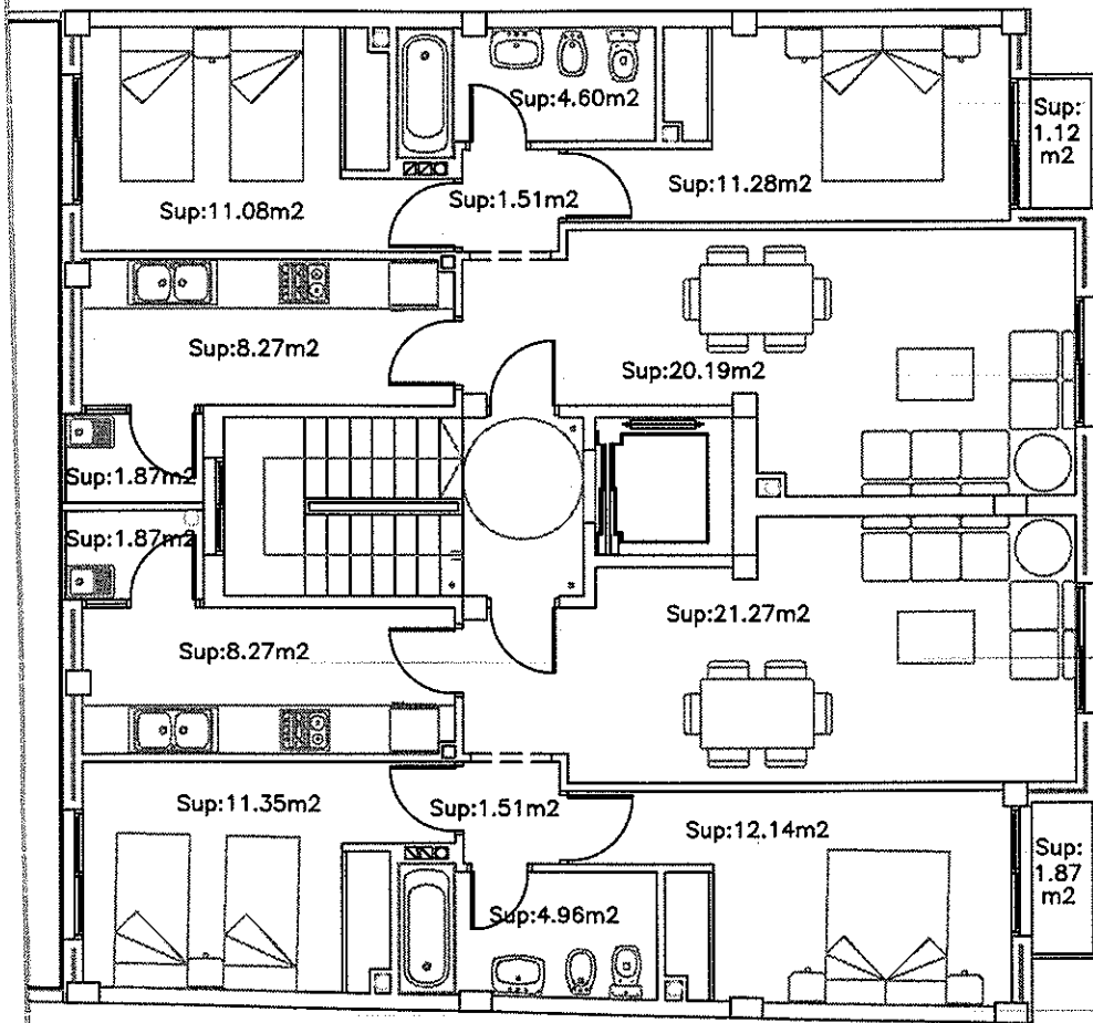
PLANTA SEGUNDA
